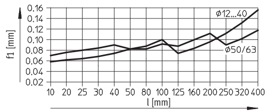
DFM-N-KF con 2 apoyos por barra de guía
