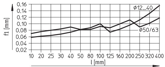
DFM-N-GF con 2 apoyos por barra de guía
